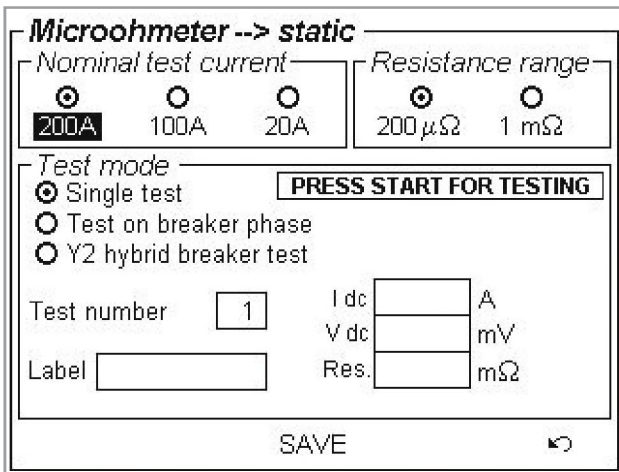
Microhmmeter display
