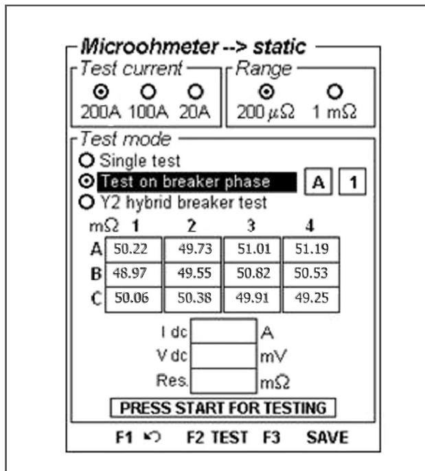
Microhmmeter display
